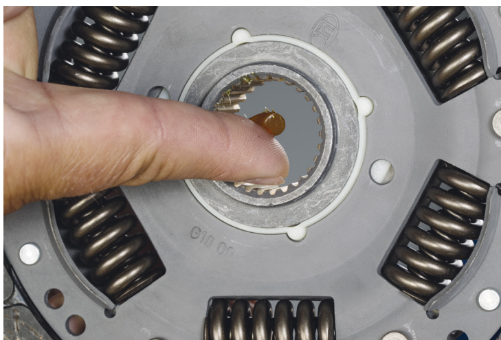
Рисунок 1: Смазка шлицов ступицы.
